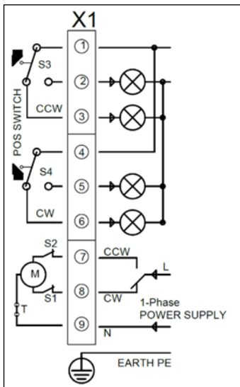
Abbildung 10: Anschlussplan
