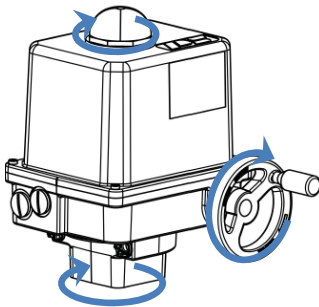
Abbildung 4: Handbetätigung
